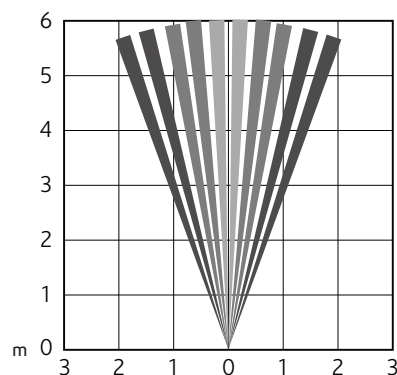
VISTA SUPERIORE
