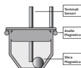
MECCANISMO INTERNO
